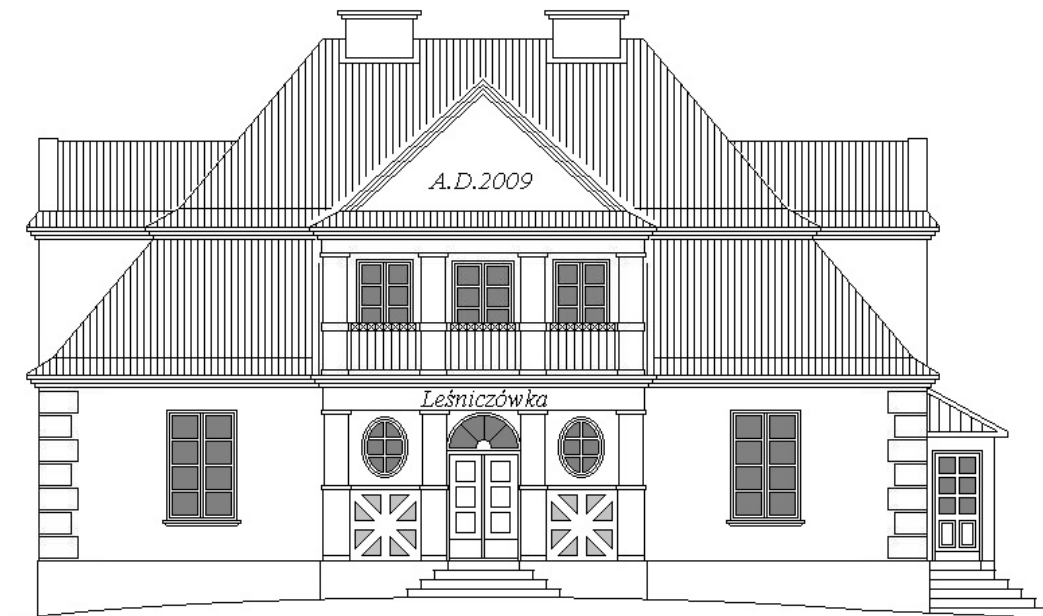
elewacja frontowa
