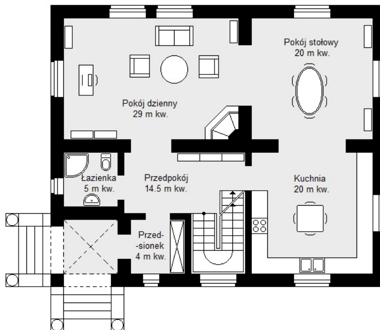
rzut parteru
