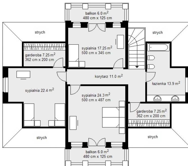
rzut poddasza
