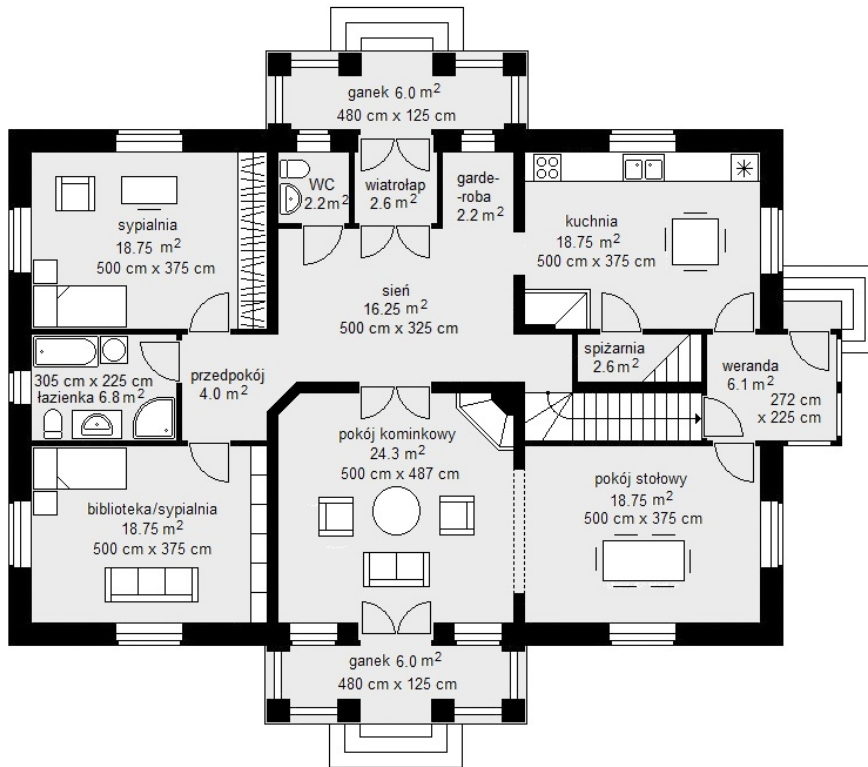
rzut parteru
