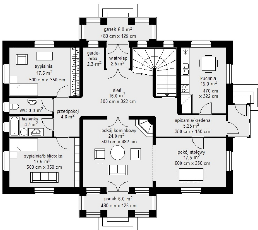
rzut parteru
