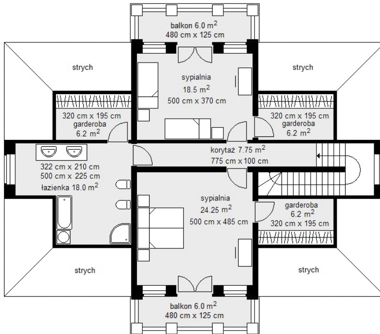
rzut poddasza
