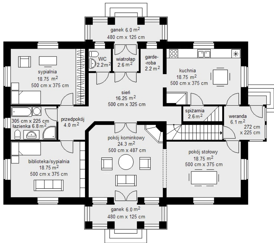
rzut parteru
