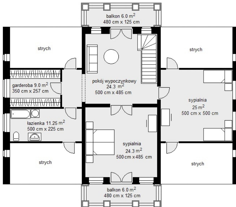
rzut poddasza
