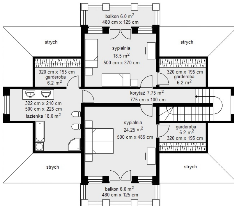
rzut poddasza
